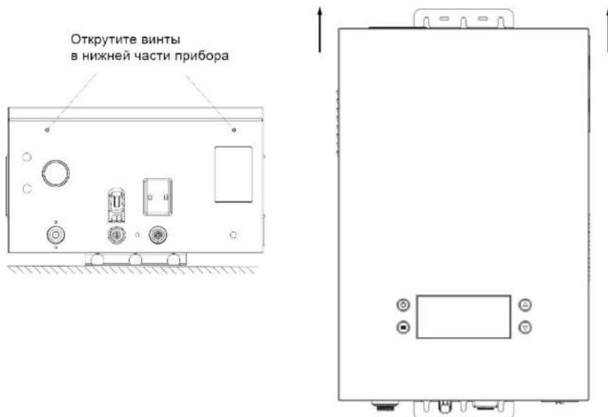
Рис. 7. Демонтаж лицевой панели
