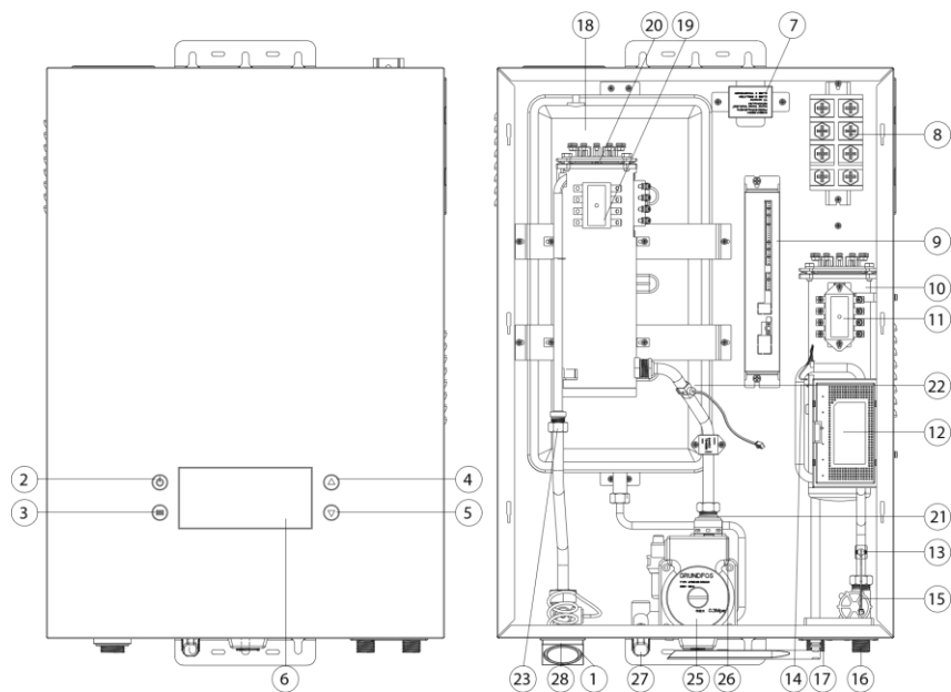
Рис. 1. Конструкция изделия
