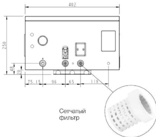
Рис. 13. Сетчатый фильтр
