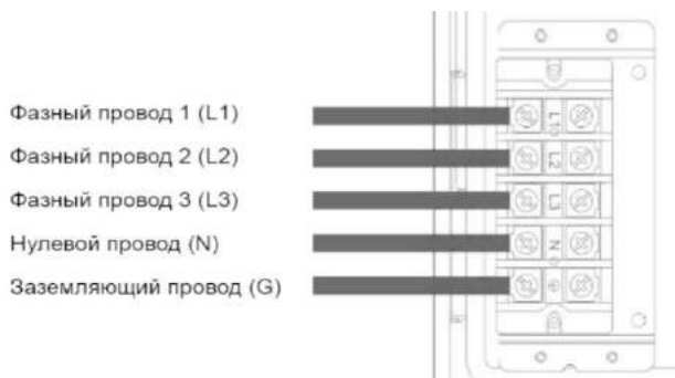
Рис.9. Подключение прибора
