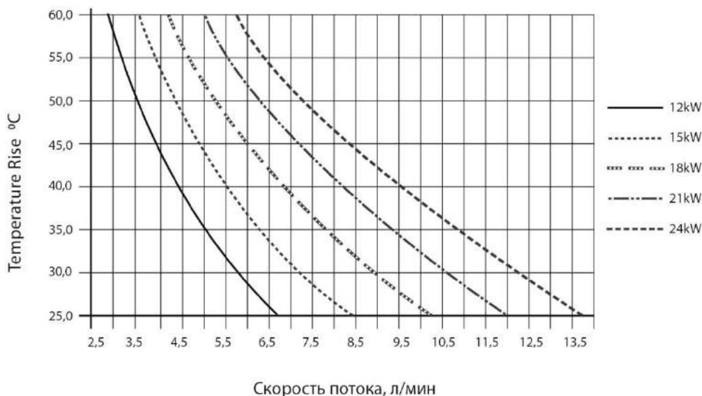
Рис. 4. График производительности системы ГВС
