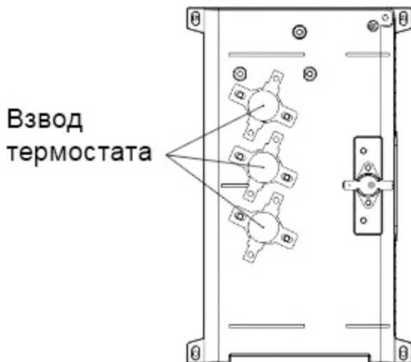
Рис. 26. Ручное восстановление термостатов
