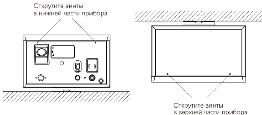
Рис. 7. Демонтаж лицевой панели
