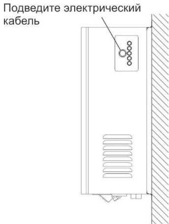
Рис. 9. Расположение панели вывода электрического кабеля
