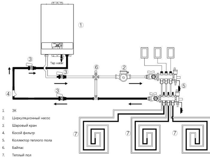
Рис. 14. Схема подключения «ЭК + Теплый пол».
