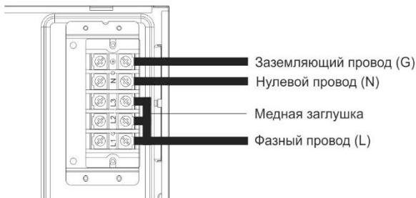
Рис 10. Однофазное подключение прибора
