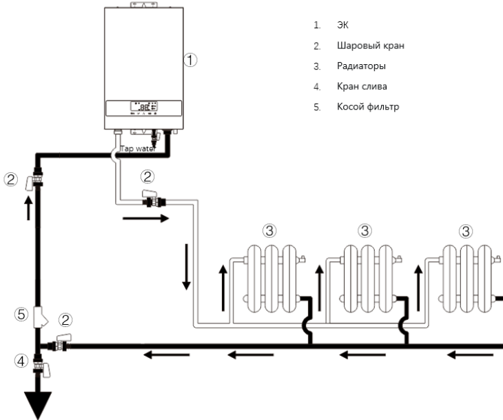
Рис. 13. Схема подключения «ЭК + Радиаторы».
