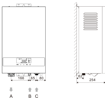
Рис. 6. Присоединительные размеры
