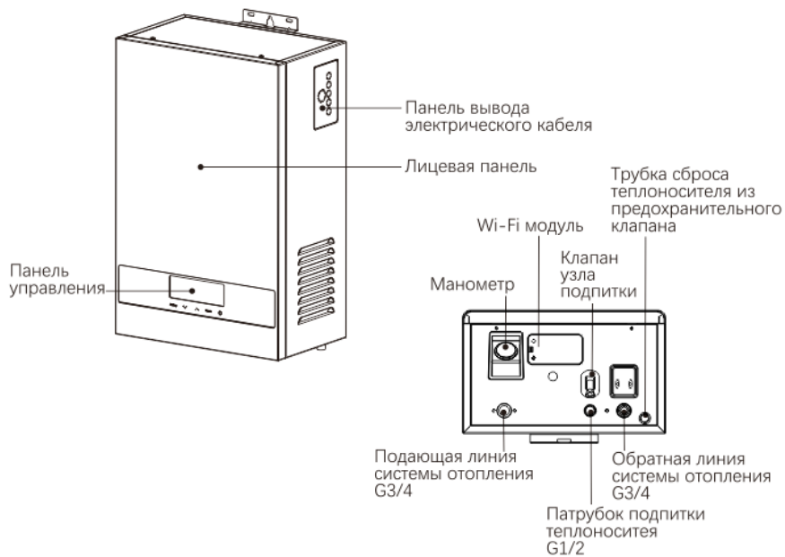
Рис. 1. Конструкция изделия
