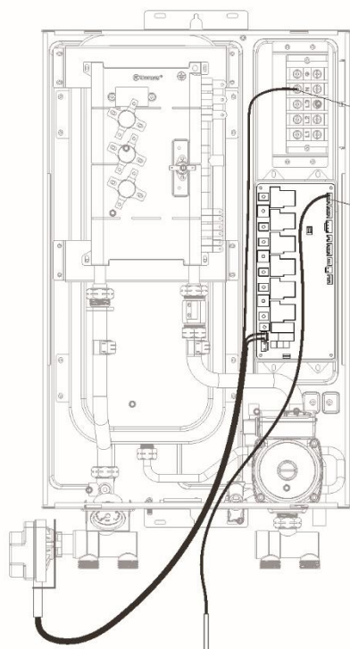
Рис. 18. Подключение датчика бойлера
