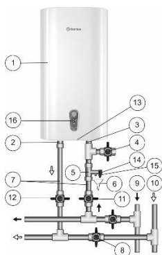
Рисунок 1. Схема подключения ЭВН к водопроводу в вертикальном положении
