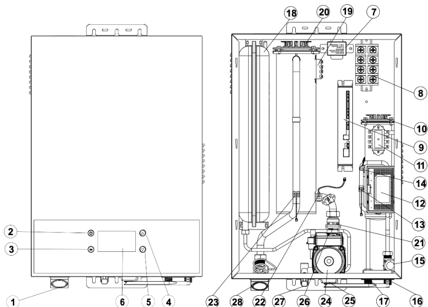
Рис. 1. Конструкция изделия
