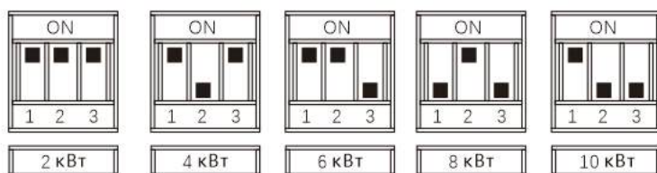
Рис. 11. Положение рычагов переключателя мощности.
