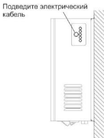
Рис. 12. Расположение панели вывода электрического кабеля
