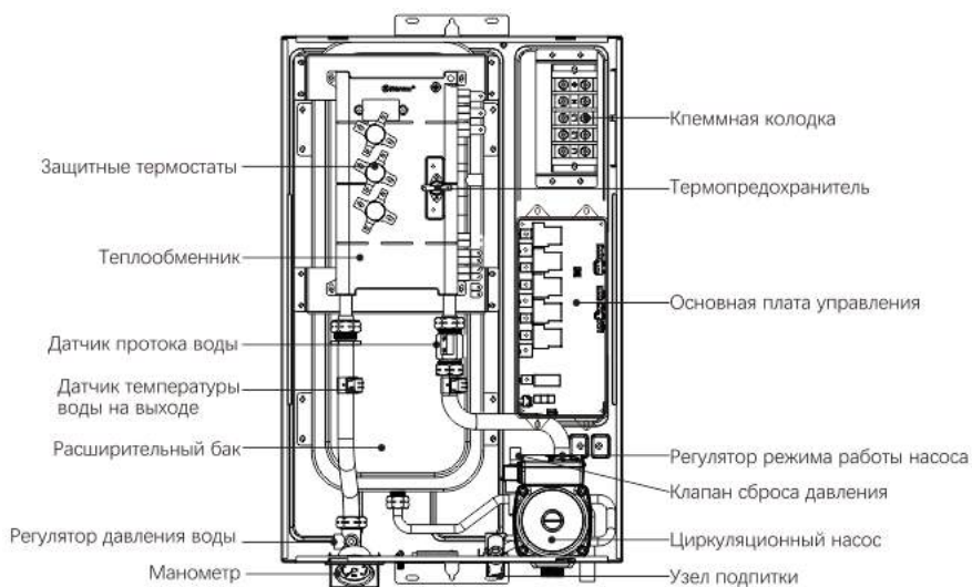
Рис. 1. Конструкция изделия
