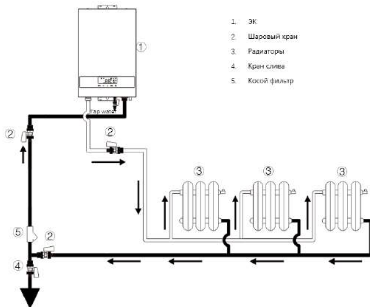
Рис. 4. Схема подключения «радиаторы + ЭК».
