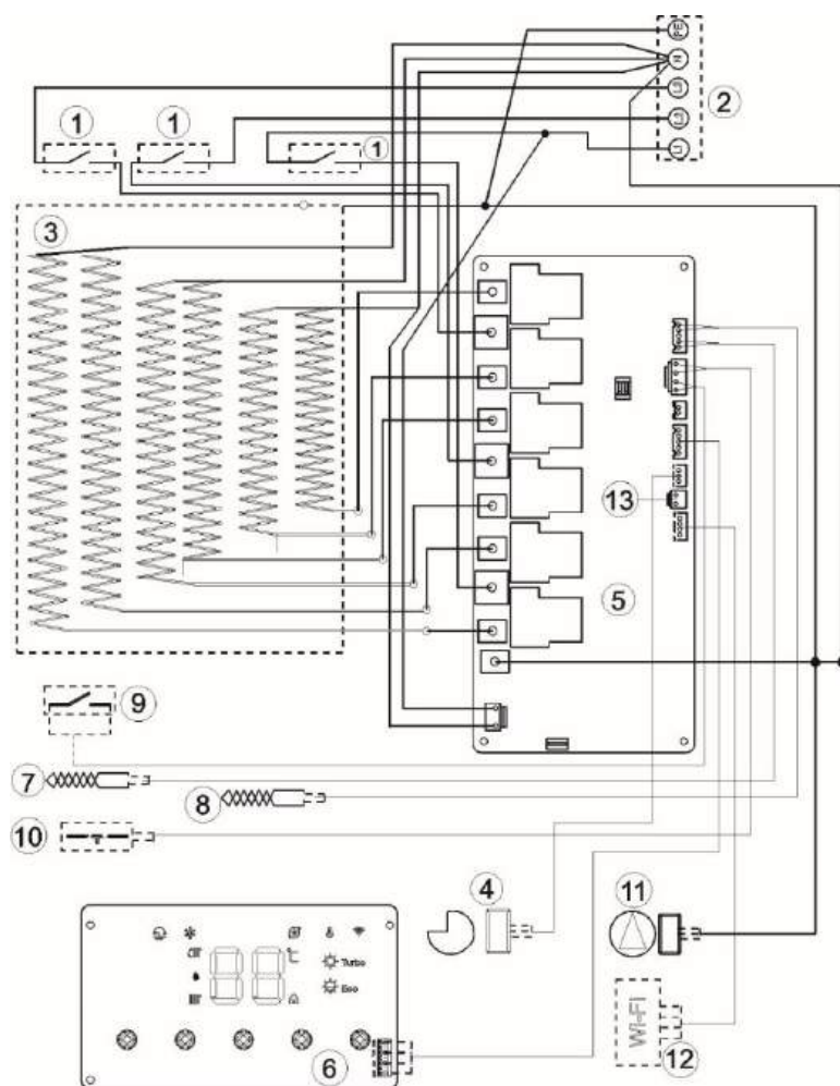
Рис. 17. Электрическая схема THERMEX Avior 10 Wi-Fi
