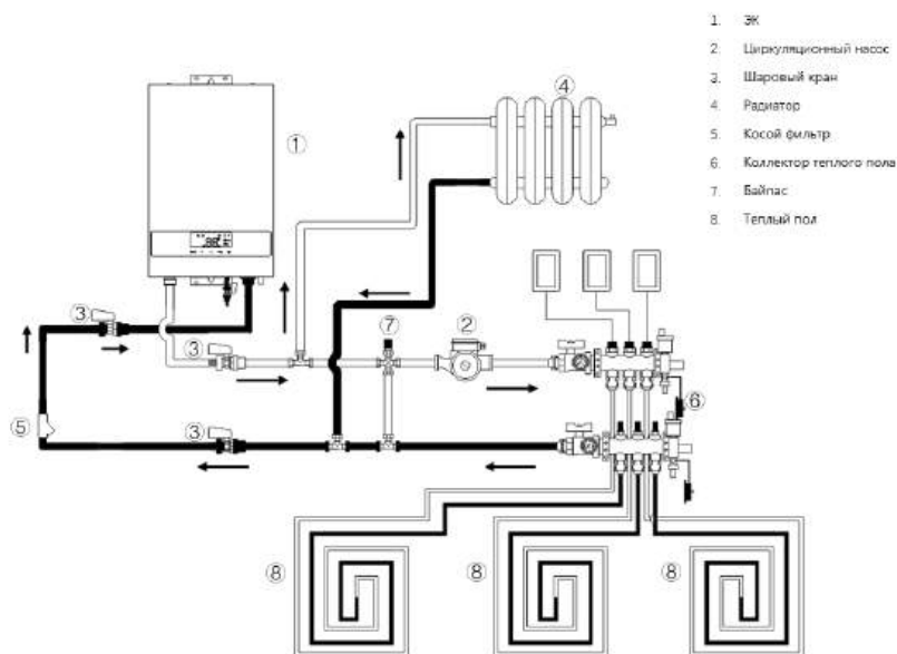
Рис. 6. Схема подключения «ЭК + Радиаторы + Теплый пол».
