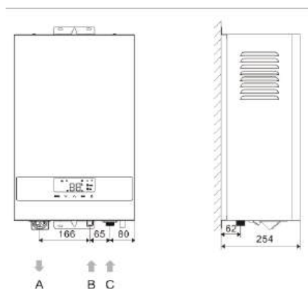
Рис. 9. Присоединительные размеры
