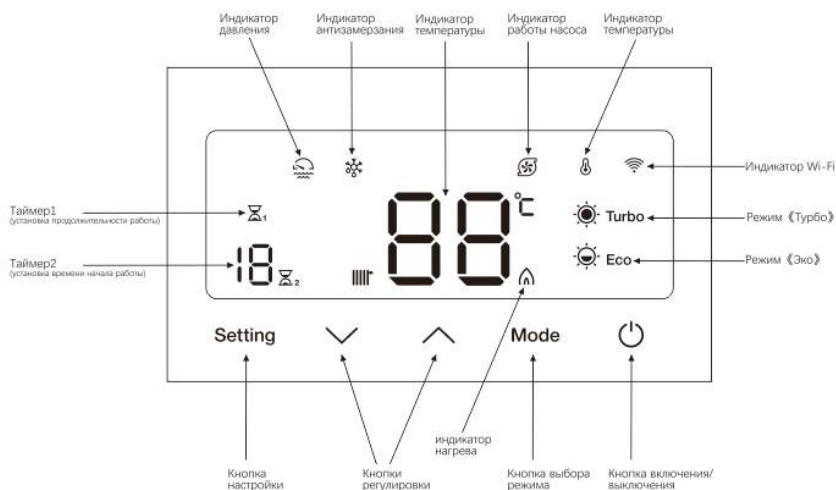
Рис. 3. Панель управления
